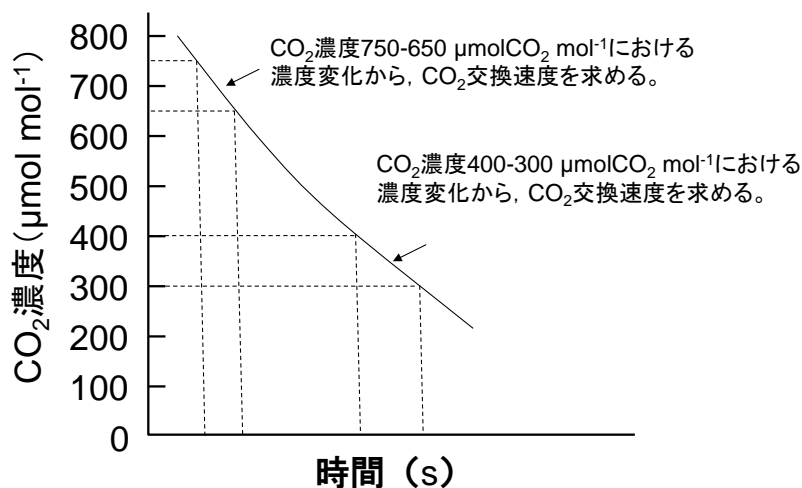
図 7 それぞれの濃度での \text{CO}_2 交換速度の求め方
